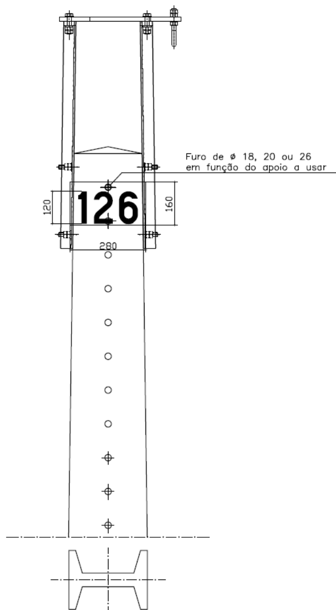
PLACA SINALÉTICA PARA APOIS DE BETÃO
