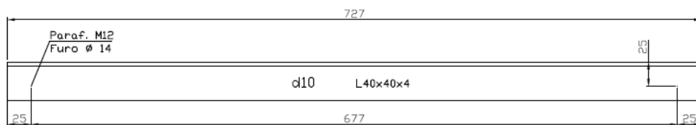
ACESSÓRIO D10-2 PEÇAS
