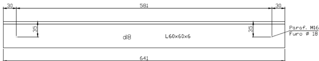
ACESSÓRIO D8—2 PEÇAS (1 Esq.+1 Dir.)
