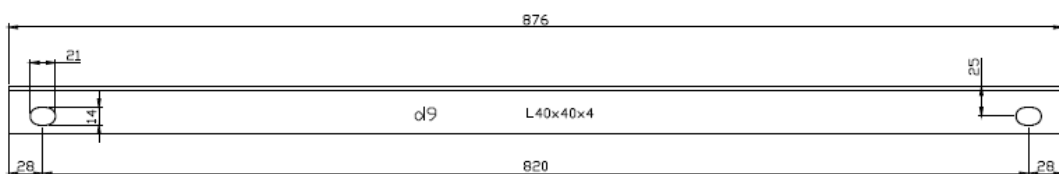
ACESSÓRIO D9—4 PEÇAS
